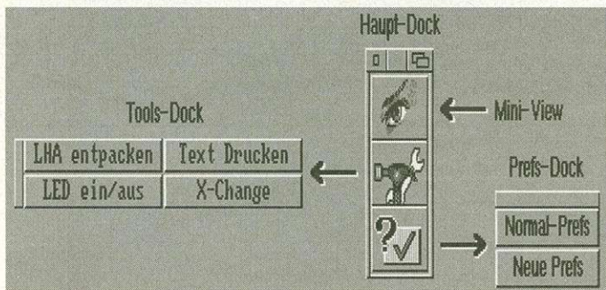
Verschachtelt: Hier sehen Sie die Zusammenhänge zwischen »Haupt-Dock«, »Tools-Dock« und »Prefs-Dock«
